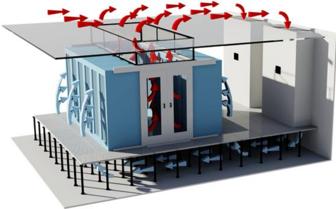
Fig. Hot Air Return
